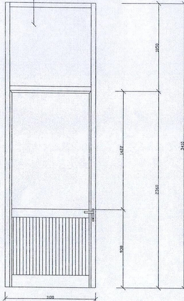
CHI TIẾT VÁCH KÍNH SỐ 3
