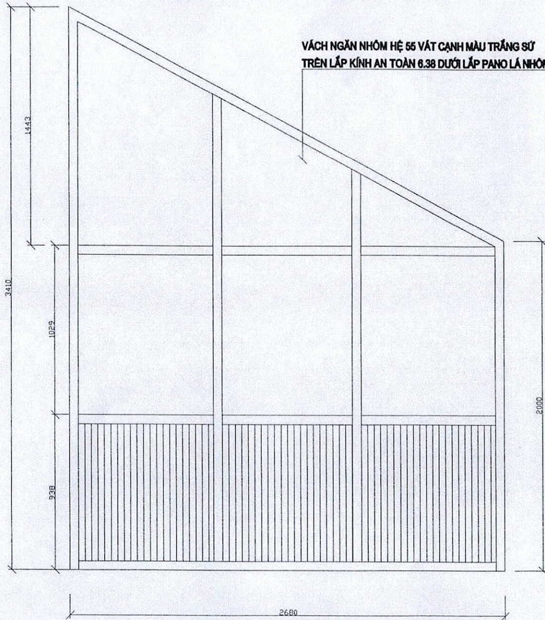
CHI TIẾT VÁCH KÍNH SỐ 3
